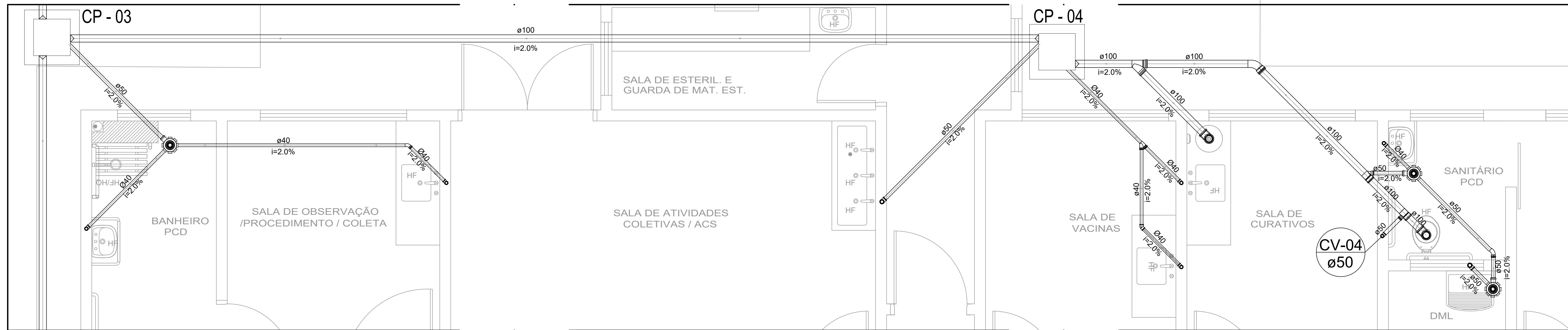
DETALHE DE ESGOTAMENTO SANITÁRIO - 02 ESCALA 1:25
