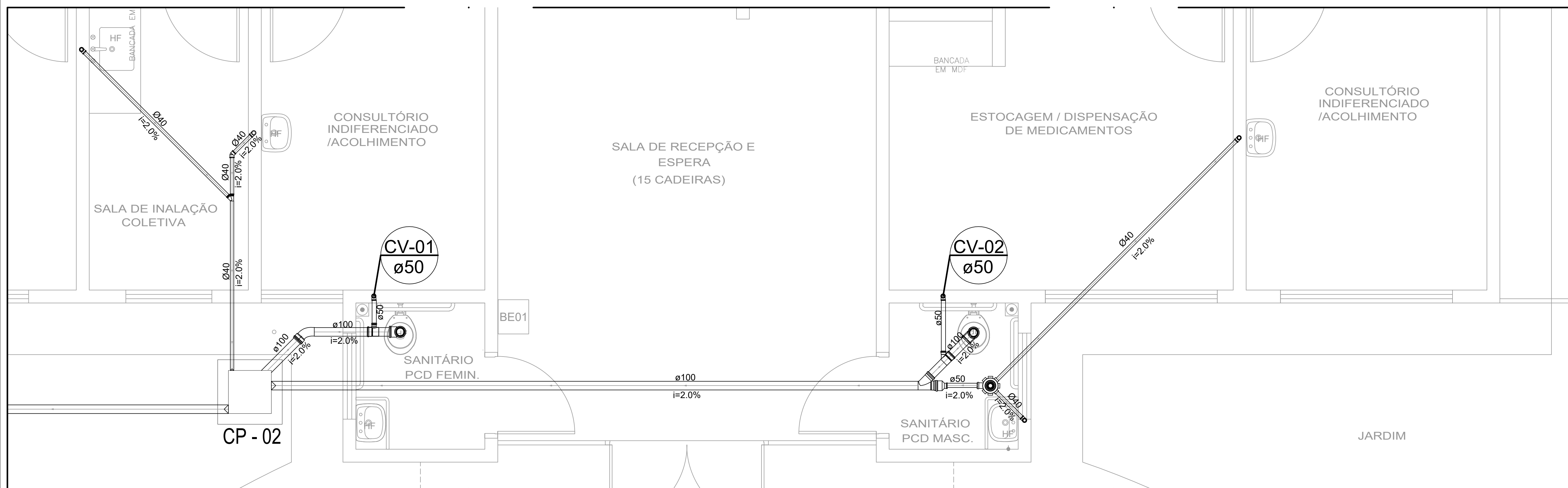
DETALHE DE ESGOTAMENTO SANITÁRIO - 03 ESCALA 1:25
